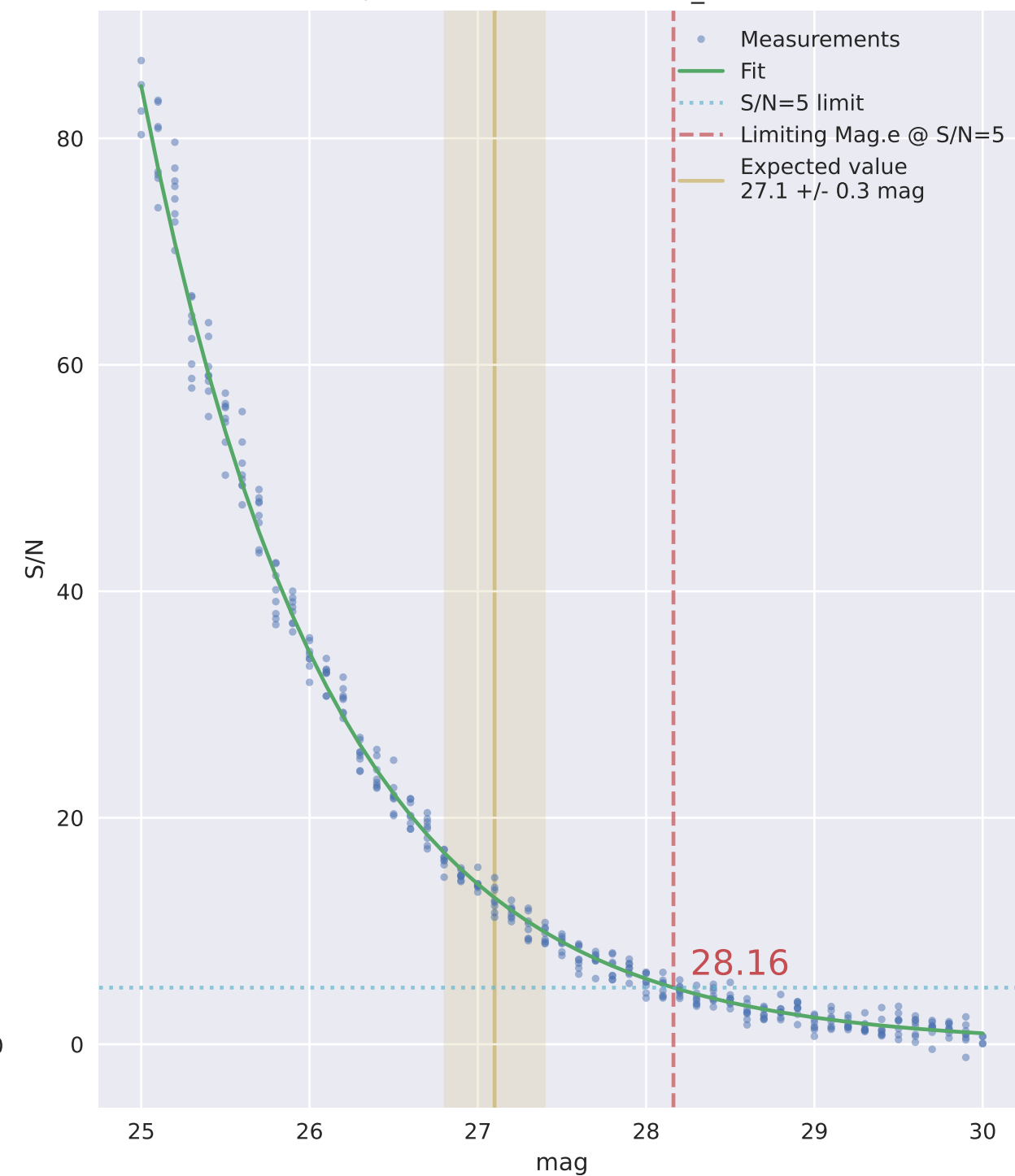
S/N for MICADO SCAO IMG_4mas
